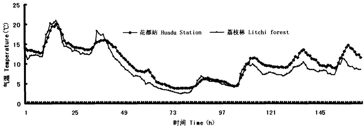
图8 冷空气过程中荔枝林冠层和花都站气温逐时变化(2002年12月23-30日)
