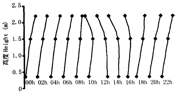
图 5 荔枝林气温垂直梯度日变化(向右为气温增大方向, 不同时间水平坐标相对独立)
