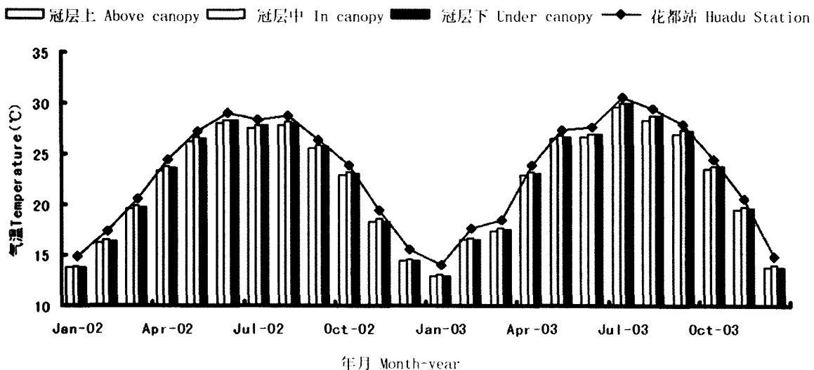
图 1 荔枝林和花都站月平均气温
