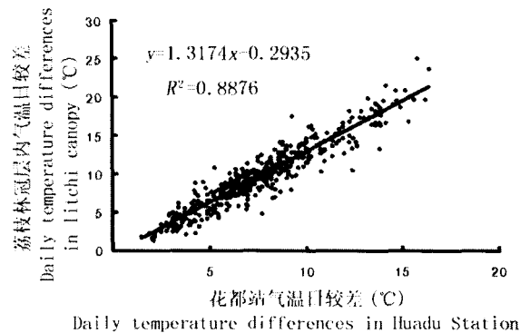
图 4 荔枝林冠层与花都站气温日较差关系
