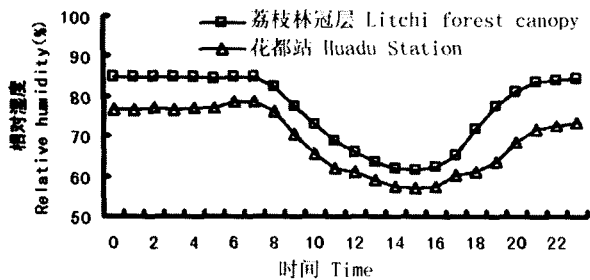
图 6 荔枝林和花都站相对湿度年平均的日变化
