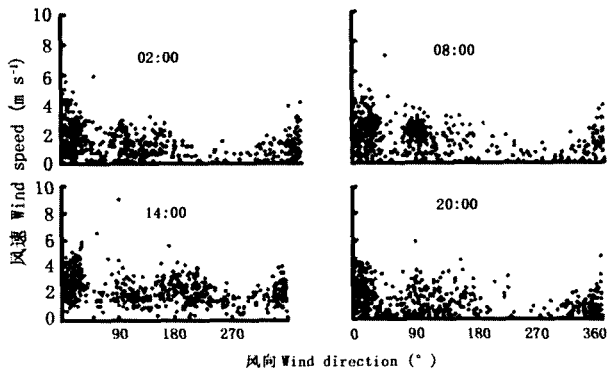
图 7 荔枝林不同时间风速、风向点聚图
