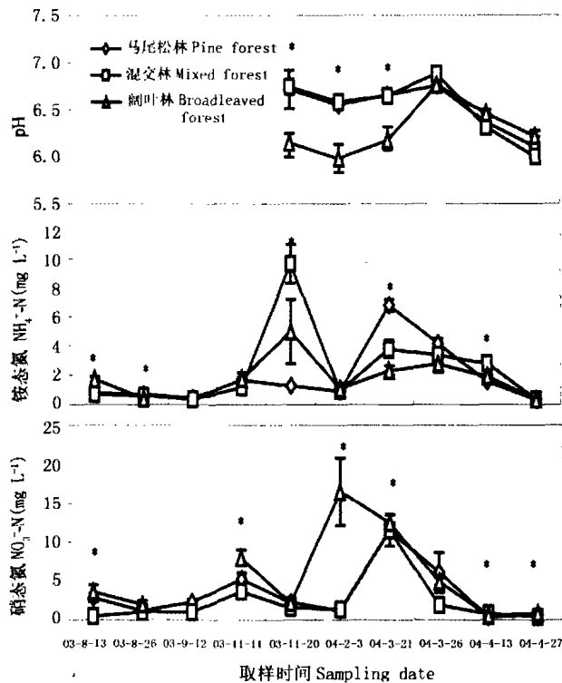
图 1 鼎湖山森林穿透雨 pH 值 and 无机氮含量
