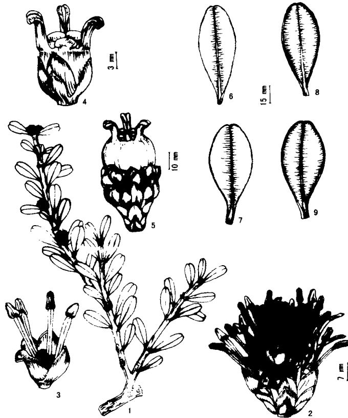
图 1 Fig. 1 潮安黄杨 Buxus chaoanensis H. G. Ye
