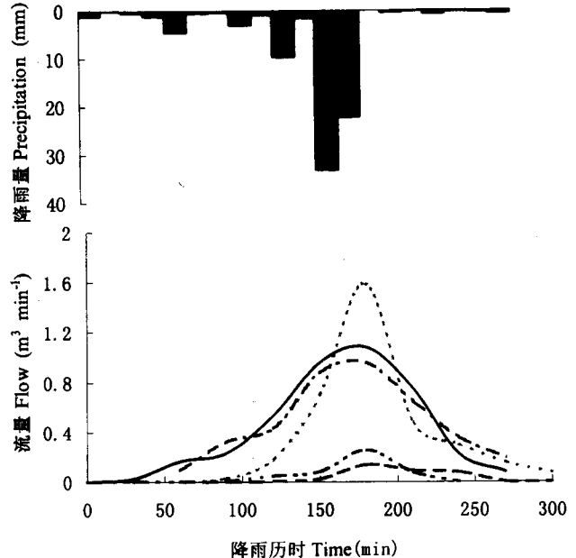
图4 5种生态系统的降雨-地表径流过程线
