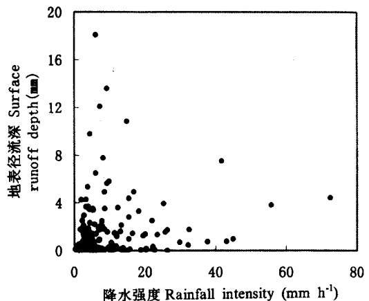
图3 豆科混交林地表径流与降水强度关系散点图
