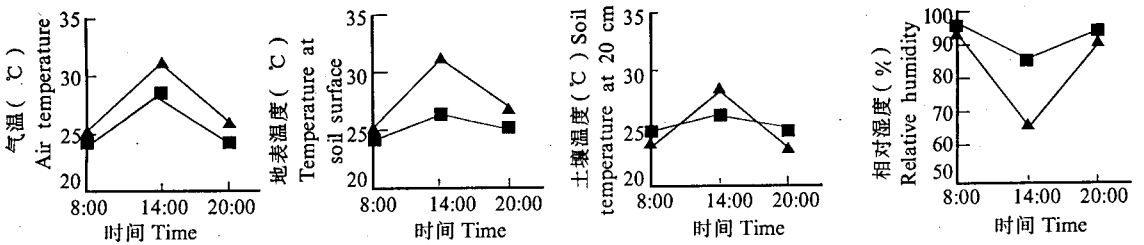
图 2 次生林 7 月各个气象要素变化曲线
